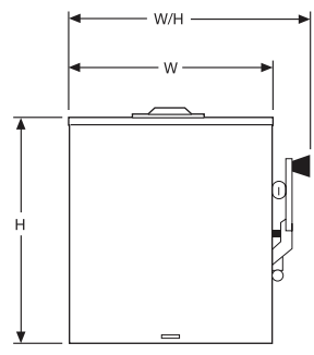
DTU-200A NEMA 3R
